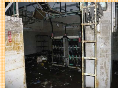
電源設備も浸水により大きく破損・損壊
