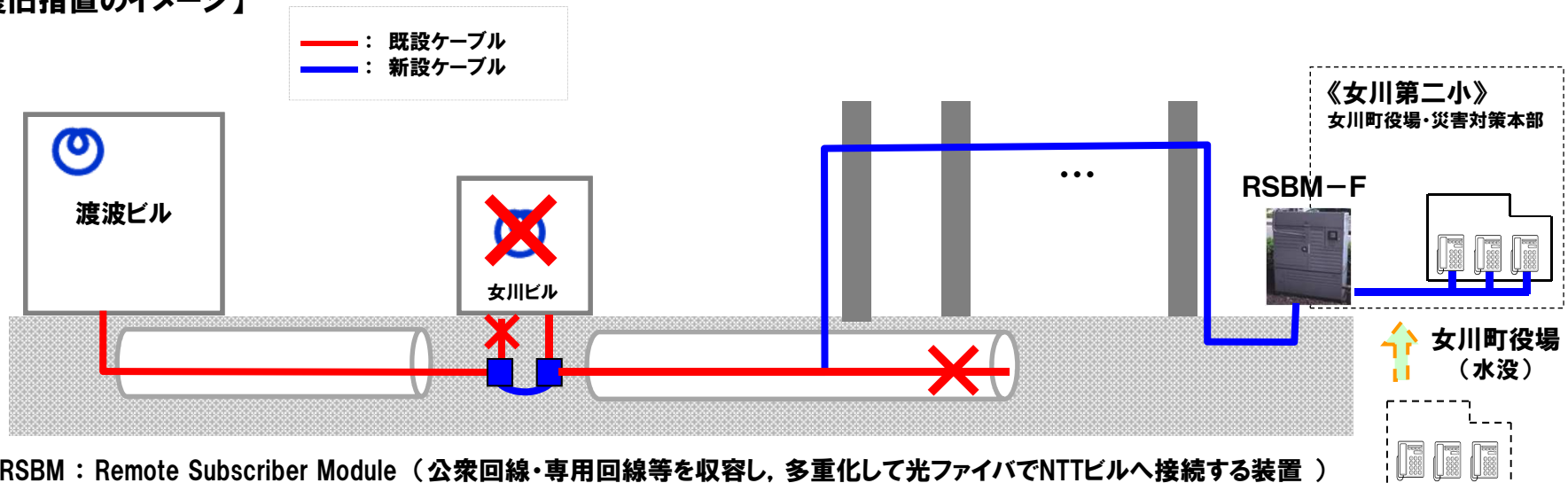
津波により周辺が水没し交換機収容ビルが大きく損壊
